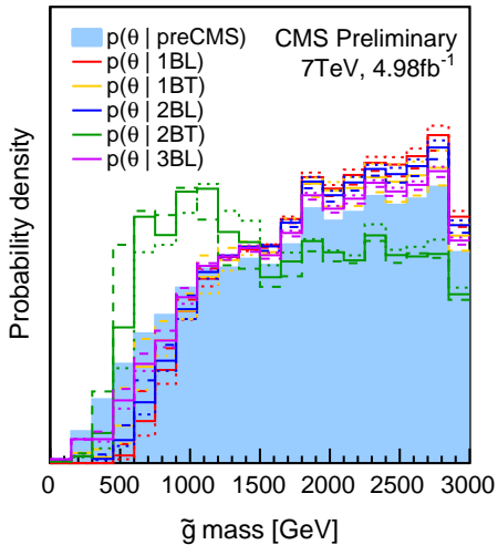
p(\theta | \text{jets} + \text{MET} + \text{b-jets})
