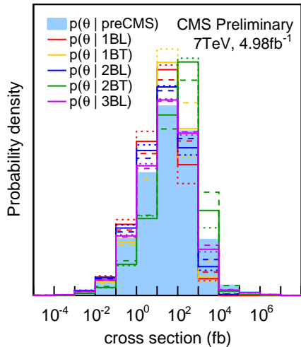
p(\theta | \text{jets} + \text{MET} + \text{b-jets})
