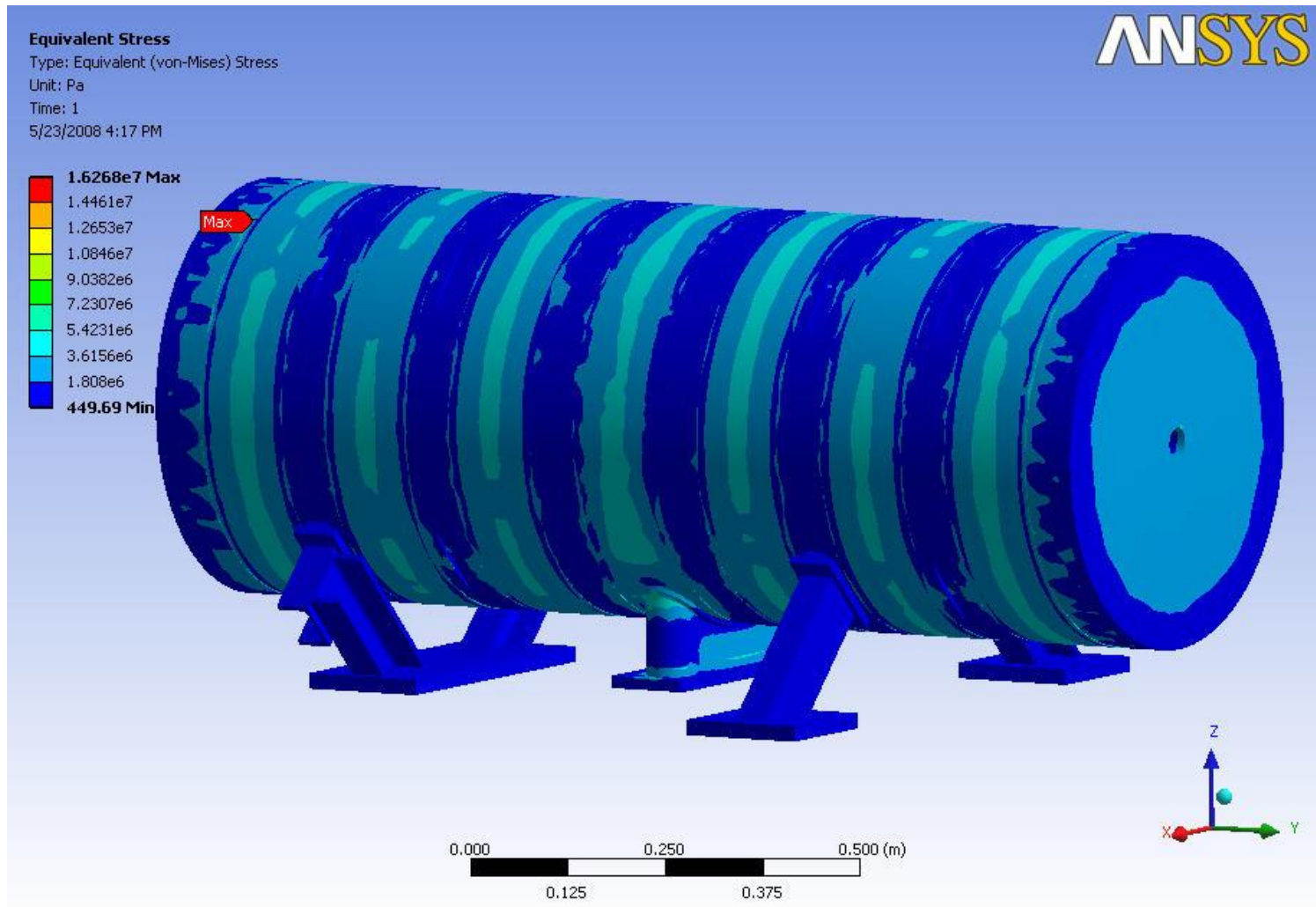
PIMS VON MISES STRESS TRUE SCALE
