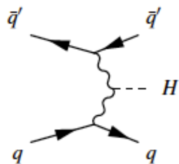
(b) VBF
