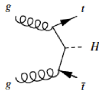
(d) t\bar{t}H
