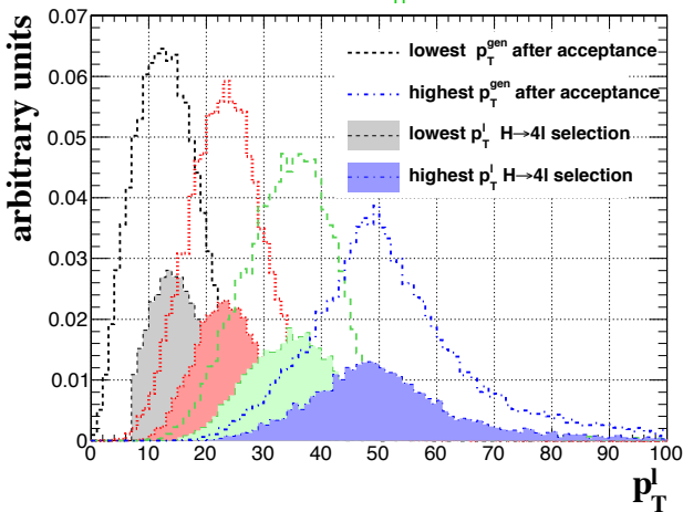
H \rightarrow ZZ^* \rightarrow 4e , m_H = 140 GeV
