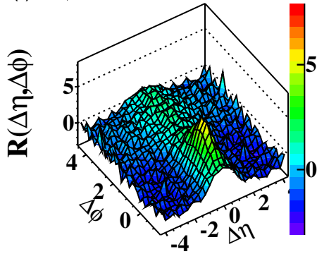
(b) CMS \sqrt{s} = 2.36\text{TeV}
