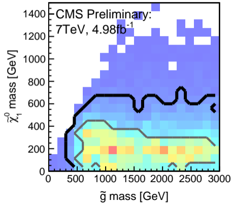
p(\theta | \text{HT + MET + bs 2BT})
