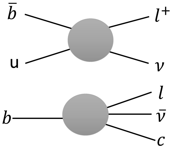
B decays
