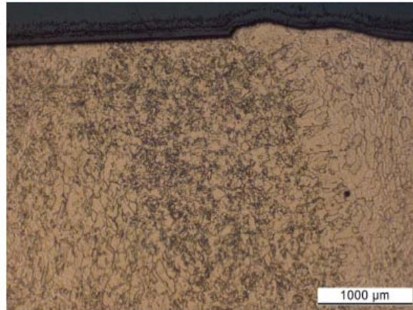
Schliffnummer: S 215 Vergrößerung: 16 : 1
