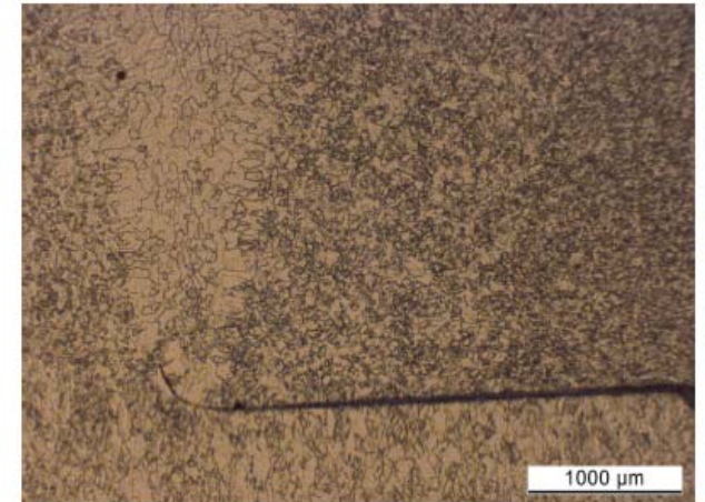
Schliffnummer: S 215 Vergrößerung: 16 : 1
